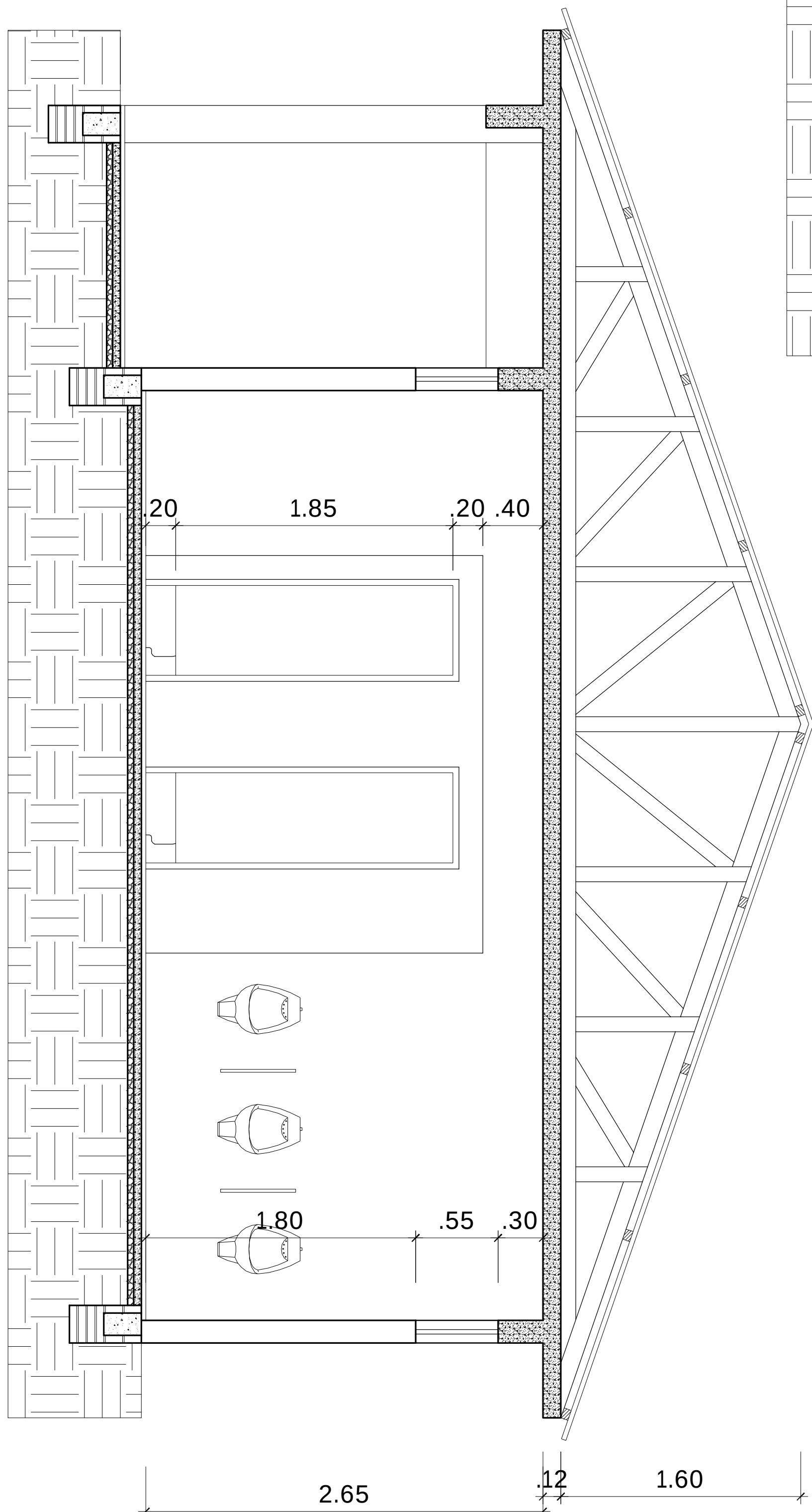
Corte B-B
