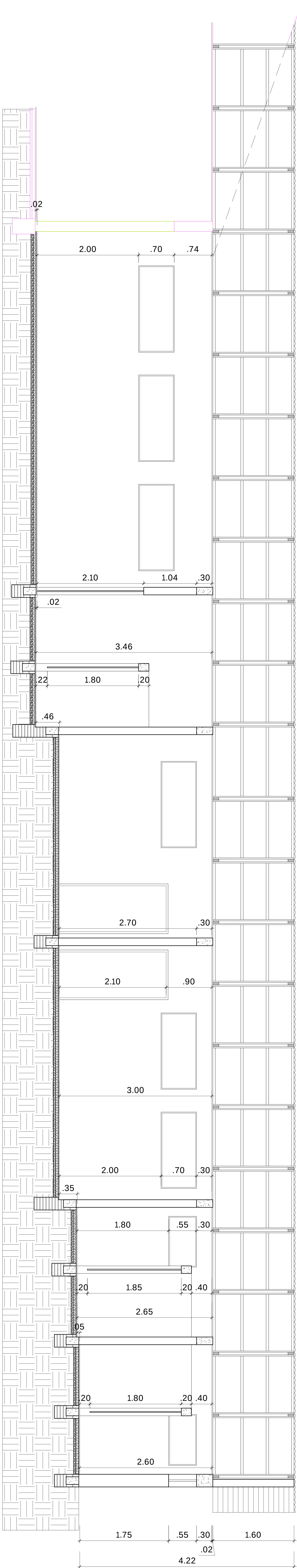
Corte A-A
